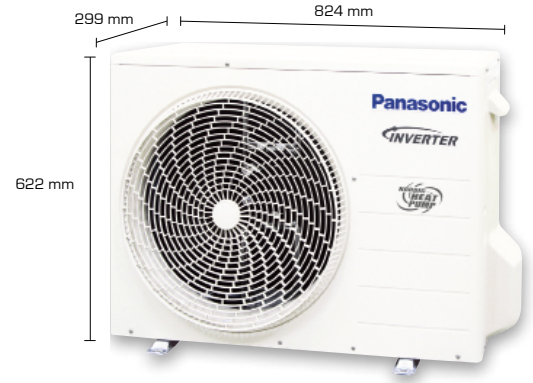
Ulkoyksikkö
